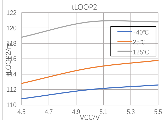
图 7-10 显性状态到隐性状态环路延时
