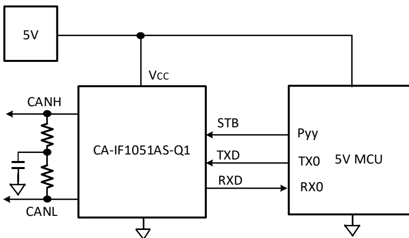
图 10-2 CA-IF1051AS-Q1 CAN 总线典型应用电路
