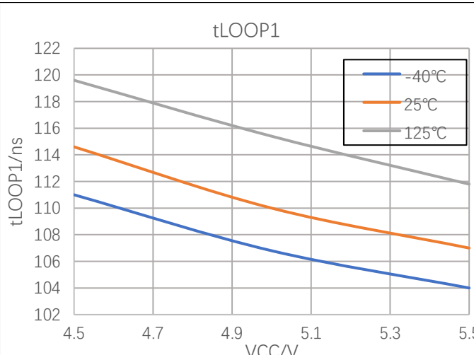
图 7-9 隐性状态到显性状态环路延时
