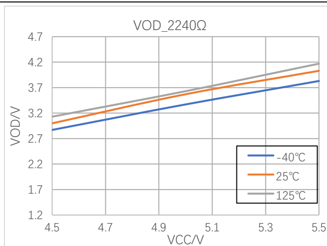
图 7-8 2240Ω 负载下差分输出电压
