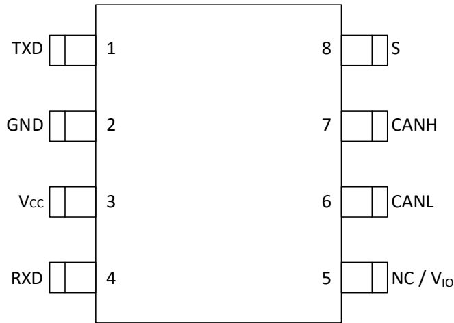
图 6-1 CA-IF1051AS-Q1 /CA-IF1051AVS-Q1 引脚配置
