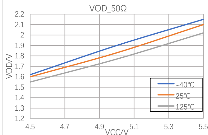
图 7-6 50Ω 负载下差分输出电压
