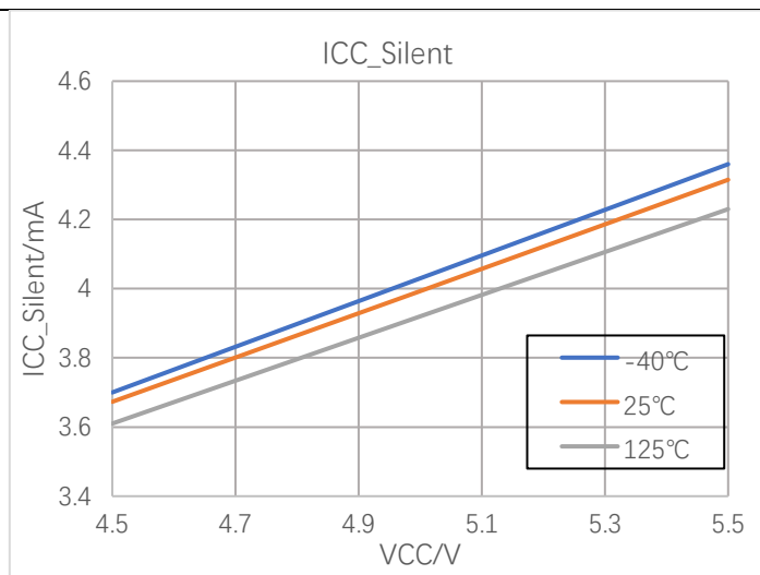
图 7-1 静音模式电流
