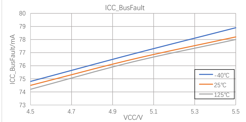
图 7-5 总线故障时电源电流
