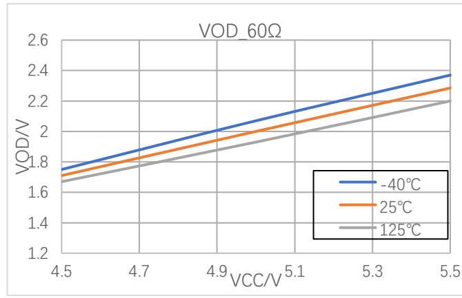
图 7-7 60Ω 负载下差分输出电压
