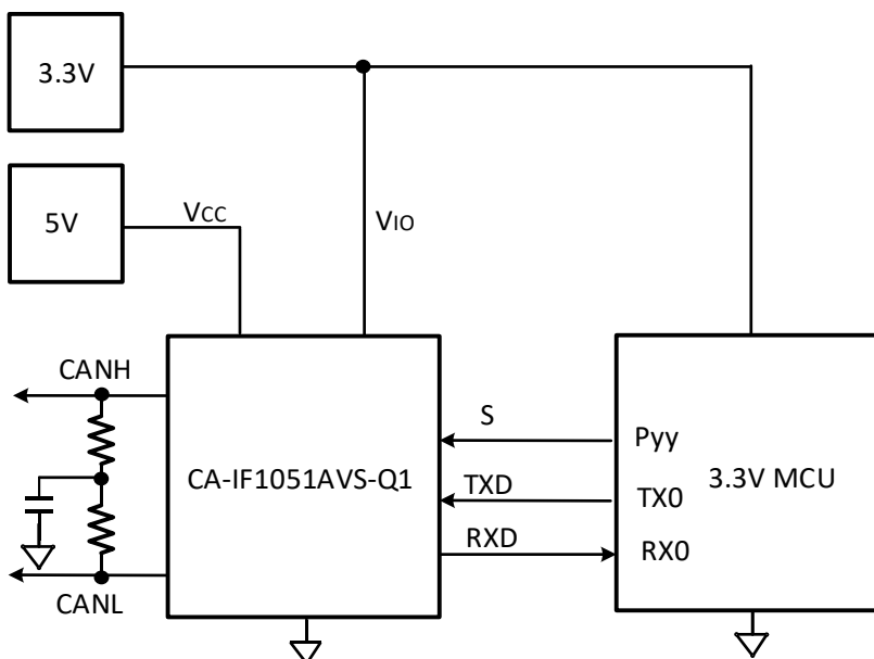
图 10-1 CA-IF1051AVS-Q1 CAN 总线典型应用电路
