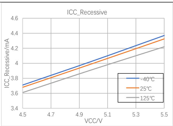
图 7-2 隐性状态电流
